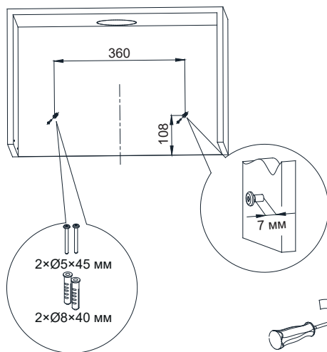
Рис. 56. Встановлення витяжки – кріплення до бічних стінок шафи
