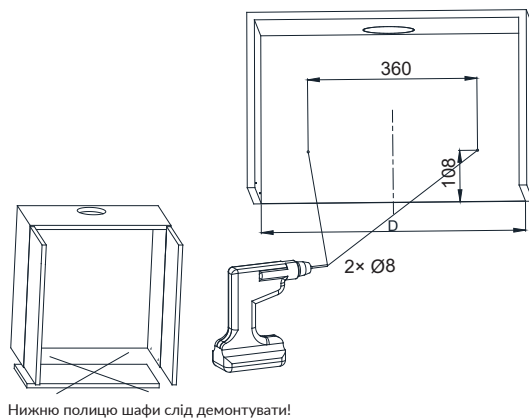
Рис. 6а. Встановлення витяжки на задню стінку шафи
