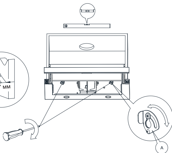
Рис. 6в. Встановлення витяжки на задню стінку шафи
