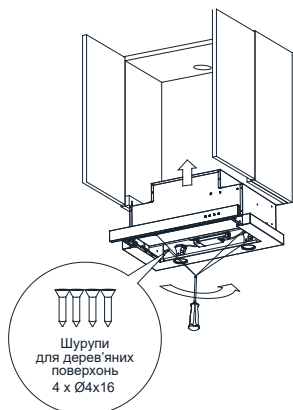
Рис. 56. Встановлення витяжки – кріплення до бічних стінок шафи
