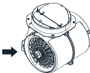
Рис. 8. б) встановлення зворотного клапану на двигун
