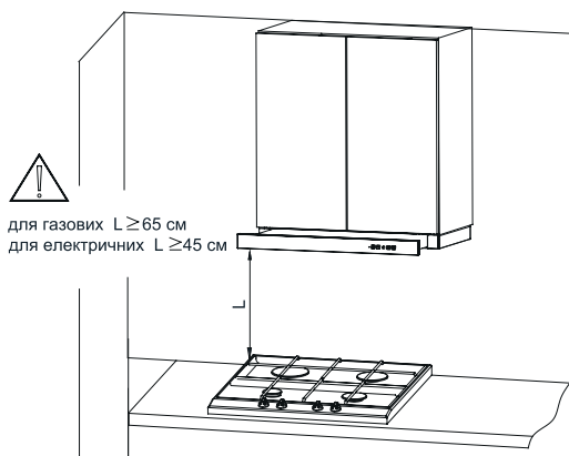
Рис. 3. Рекомендована відстань від плити
