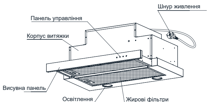
Рис. 1. Загальний вид витяжки
