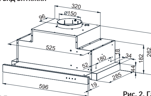
Рис. 2. Габаритні розміри
